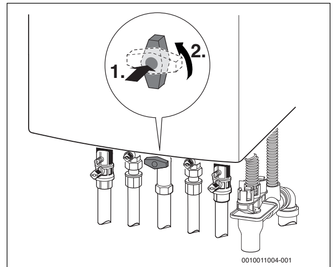
Σχ. 2 Άνοιγμα βάνας αερίου
