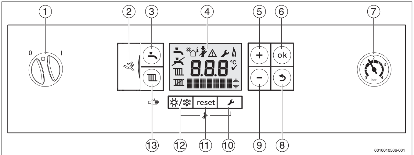
Σχ. 1 Πεδίο χειρισμού με ανοιχτό κάλυμμα πεδίου χειρισμού
